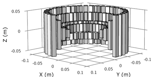
Abb. 1: Permanentmagnetaufbau für die Erzeugung der magnetischen Felder.
