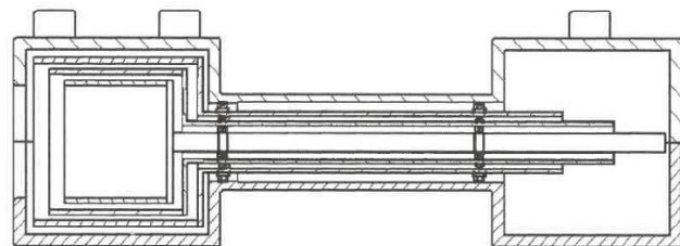
Abb. 2: CAD Zeichnung des entwickelten Designs für den Aufbau des schnell rotierenden MPI Systems.
